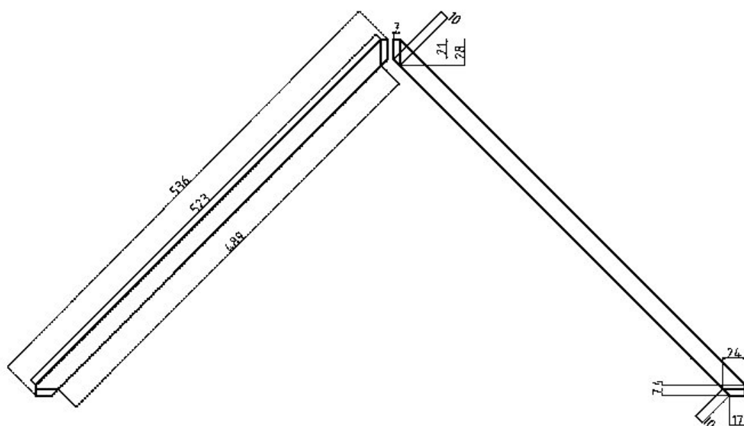
ferme X 4 arbaletrier
