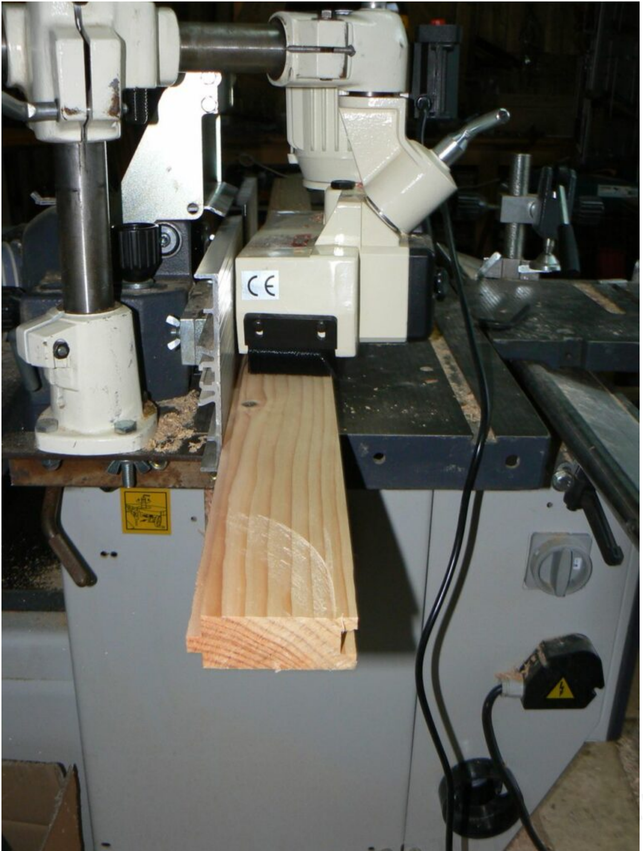
Le mange doigt de bricoleur distrait ou la toupie et sa fraise a rainurer
